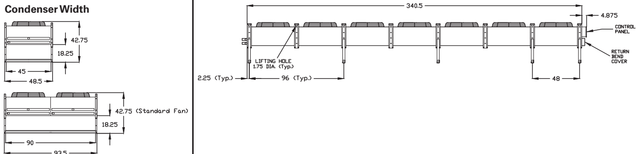
Condenser Width
