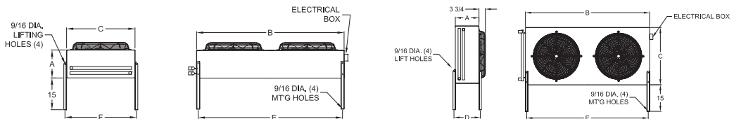
DRAWING - 2 FAN
